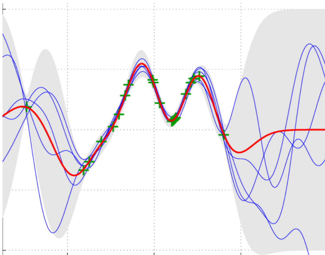
Rysunek 4.8: Wizualizacja procesu gaussowskiego. Zielonymi plusami zaznaczono obserwacje, niebieskie krzywe to poprzednie przekonania a posteriori , zaś czerwona krzywa to ich średnia wartość. Zaciemniona część wykresu wyznacza niepewność modelu. Źródło: [8]
